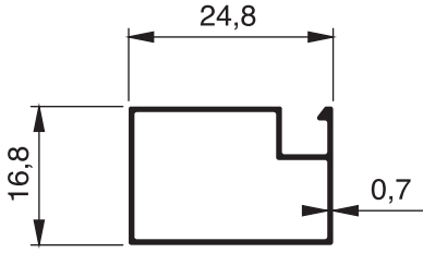
750 - 0.168 Kg/m
