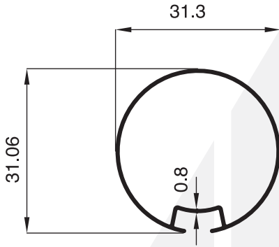
2221 - 0.231 Kg/m
