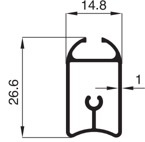
2224 - 0.259 Kg/m
