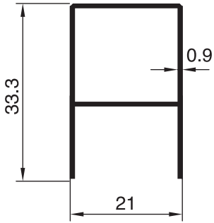
2496 - 0.256 Kg/m
