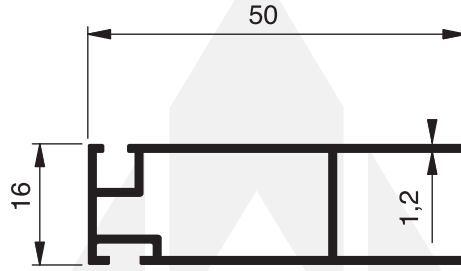
1825 - 0.437 Kg/m
