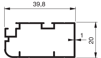
756 - 0.369 Kg/m
