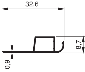
752 - 0.150 Kg/m
