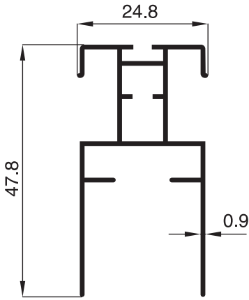
2110 - 0.416 Kg/m
