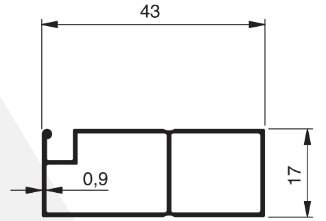
2032 - 0.373 Kg/m
