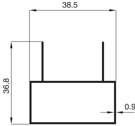
2111 - 0.359 Kg/m
