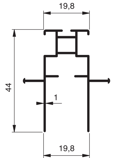
1959 - 0.435 Kg/m
