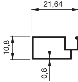
751 - 0.142 Kg/m
