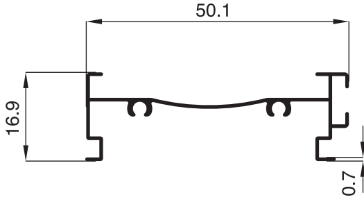
2222 - 0.238 Kg/m
