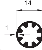
2223 - 0.194 Kg/m
