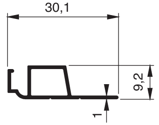
753 - 0.168 Kg/m
