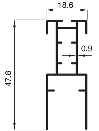
2497 - 0.381 Kg/m
