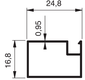
757 - 0.222 Kg/m
