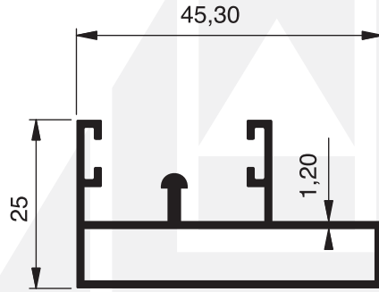
1824 - 0.545 Kg/m
