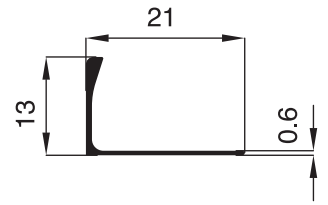
2288 - 0.073 Kg/m
