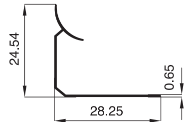
2321- 0.102 Kg/m
