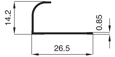
2320- 0.104 Kg/m
