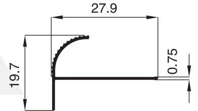
2075- 0.112 Kg/m
