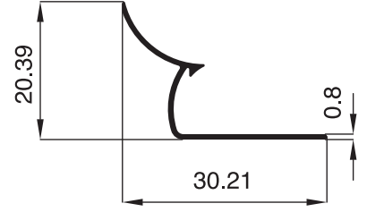
1881- 0.110 Kg/m
