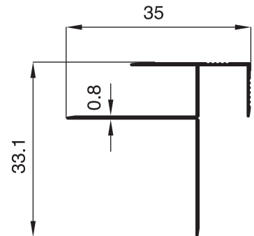
2290 - 0.190 Kg/m
