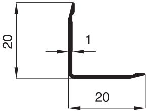
1882 - 0.102 Kg/m
