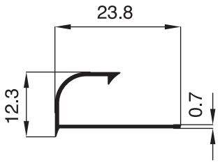
2257- 0.103 Kg/m
