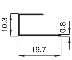
2256 - 0.087 Kg/m
