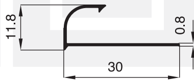
2003 - 0.108 Kg/m
