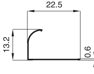
2239- 0.064 Kg/m
