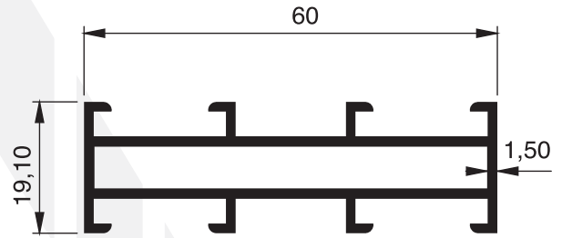
907 - 0.761 Kg/m
