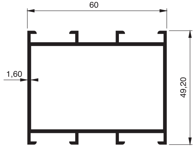
901 - 1.056 Kg/m
