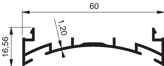
909 - 0.430 Kg/m
