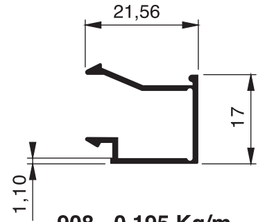
908 - 0.195 Kg/m
