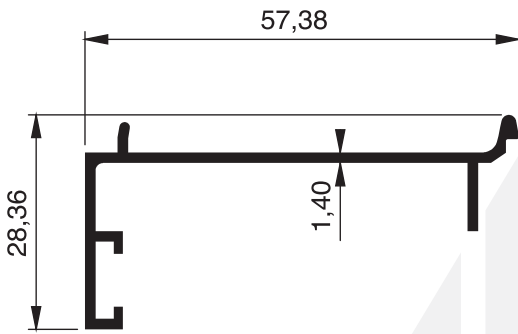
905 - 0.404 Kg/m
