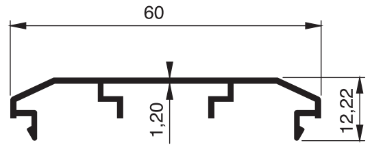
904 - 0.344 Kg/m
