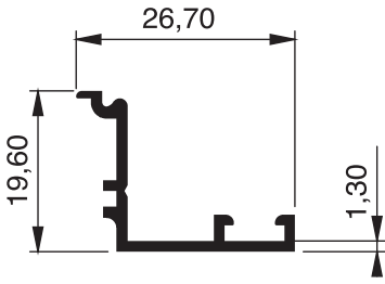
900 - 0.206 Kg/m
