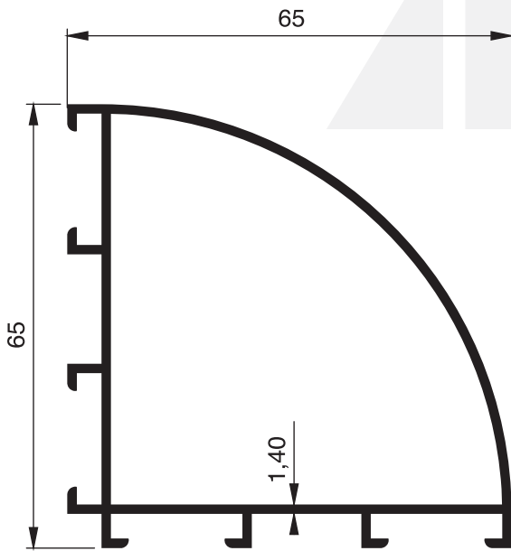
906 - 1.017 Kg/m
