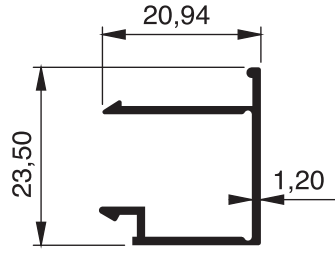
903 - 0.211 Kg/m
