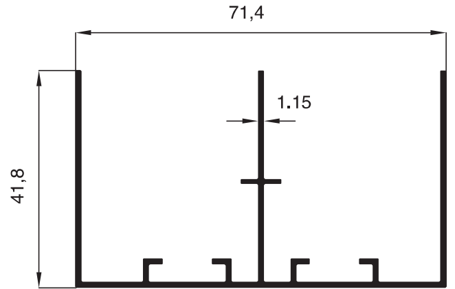
2006 - 0.710 Kg/m
