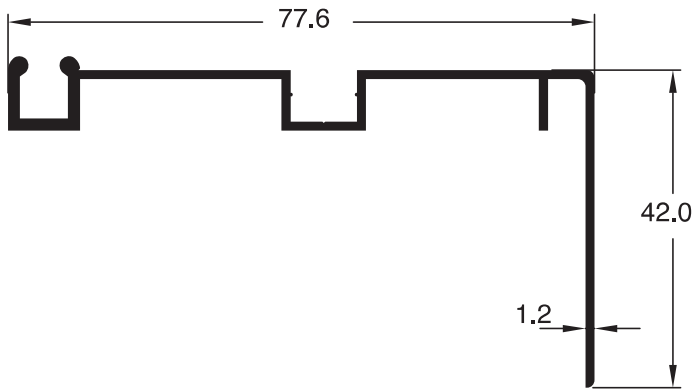
2164 - 0.542 Kg/m
