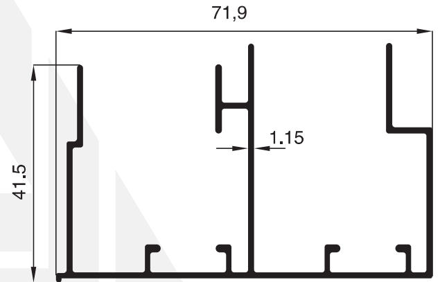
2005 - 0.800 Kg/m
