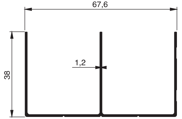
1885 - 0.572 Kg/m
