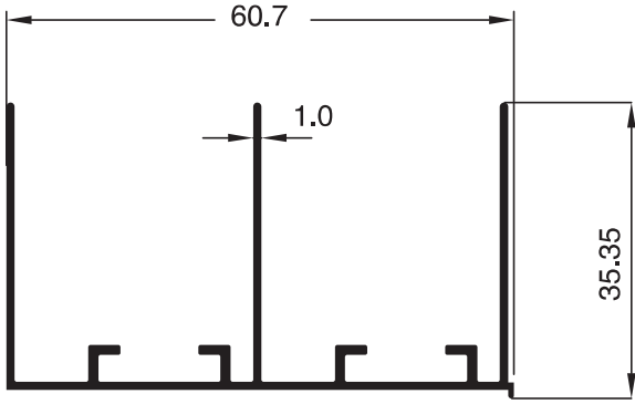
2198 - 0.530 Kg/m
