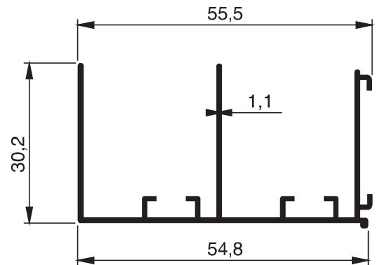
1913 - 0.519 Kg/m
