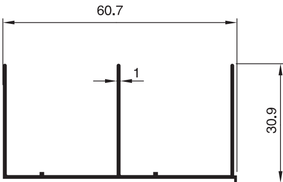
2197 - 0.406 Kg/m
