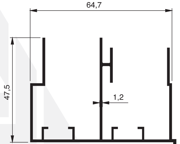
1216 - 0.860 Kg/m
