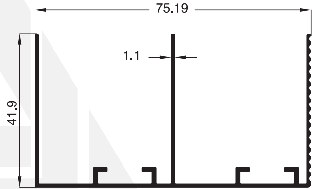
2116 - 0.678 Kg/m
