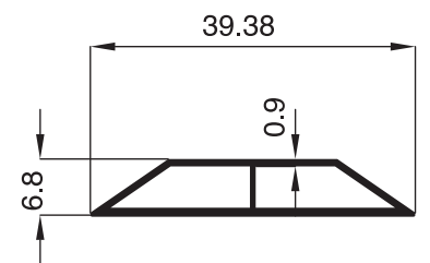
1938 - 0.191 Kg/m
