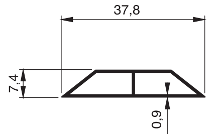
997 - 0.201 Kg/m
