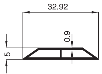
1937 - 0.164 Kg/m
