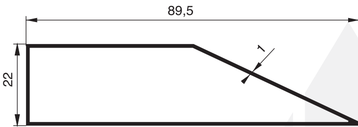
1002 - 0.550 Kg/m
