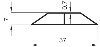
992 - 0.155 Kg/m
