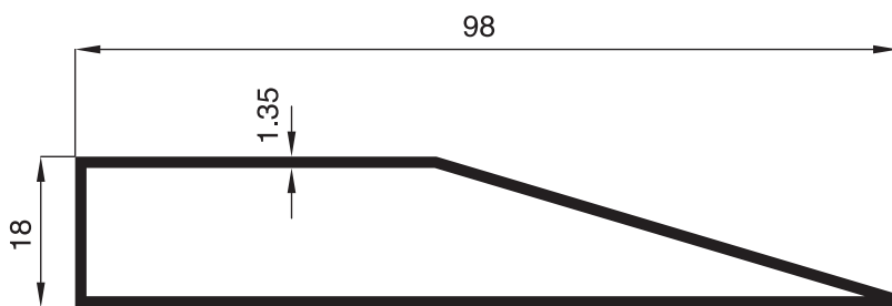
2270 - 0.775 Kg/m
