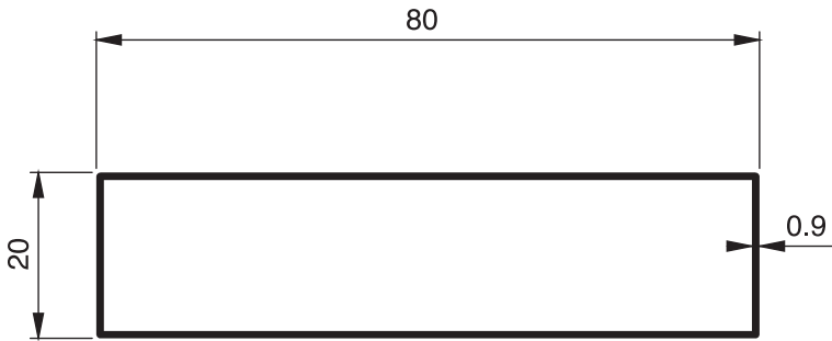
996 - 0.478 Kg/m
