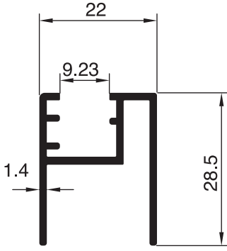
2506 - 0.372 Kg/m
