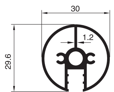
2160 - 0.568 Kg/m
