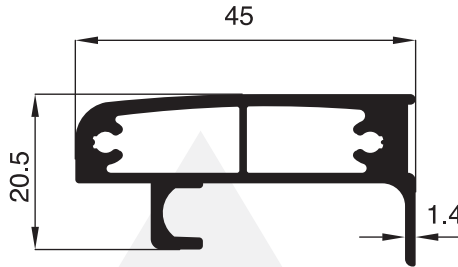
2269 - 0.739 Kg/m
