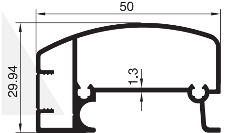
2381 - 0.691 Kg/m
