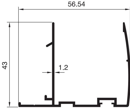
1026 - 0.530 Kg/m
