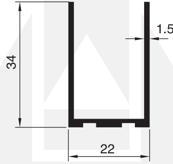
2209 - 0.374 Kg/m
