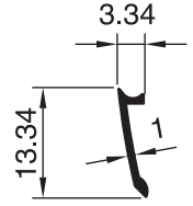
2368 - 0.044 Kg/m
