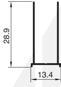
2409 - 0.150 Kg/m
