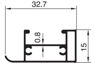
2411 - 0.264 Kg/m
