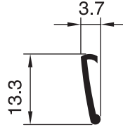
2161 - 0.051 Kg/m
