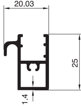
2503 - 0.356 Kg/m
