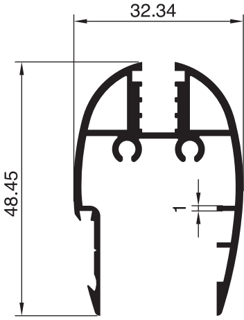
2367 - 0.765 Kg/m
