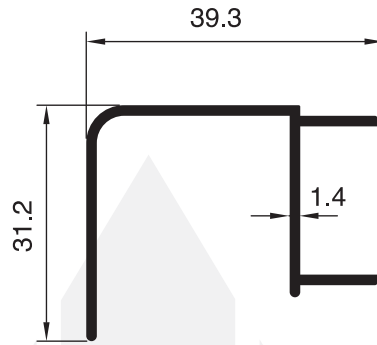
1283 - 0.385 Kg/m
