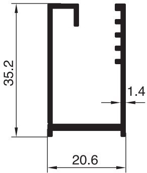
2446 - 0.433 Kg/m
