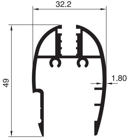
2158 - 0.775 Kg/m
