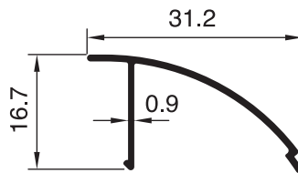
1028 - 0.140 Kg/m
