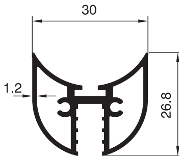
2162 - 0.545 Kg/m
