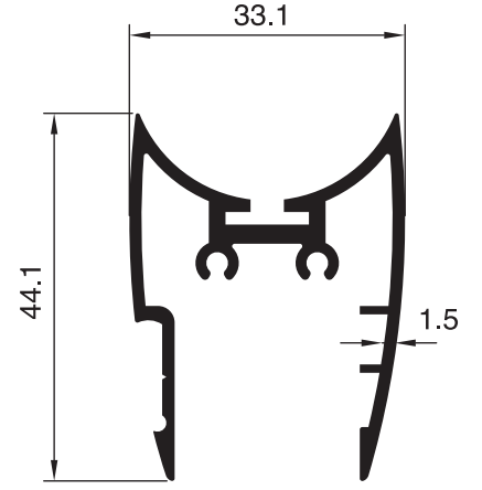
2159 - 0.710 Kg/m
