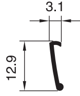
2218 - 0.045 Kg/m
