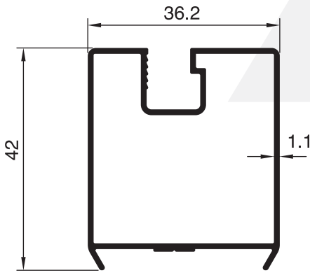
1027 - 0.544 Kg/m
