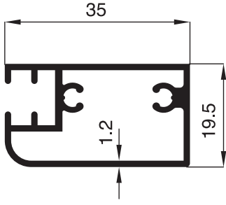
1282 - 0.481 Kg/m
