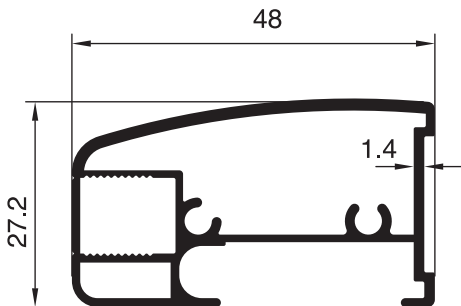
1029 - 0.705 Kg/m
