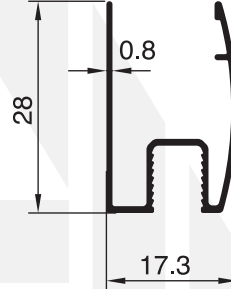
2412 - 0.202 Kg/m
