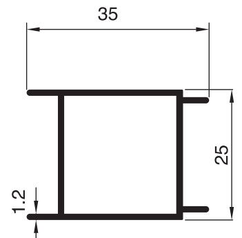
1279 - 0.379 Kg/m
