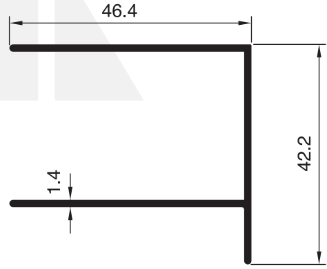
1263 - 0.500 Kg/m
