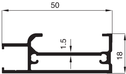
2481 - 0.600 Kg/m
