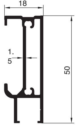
2504 - 0.600 Kg/m
