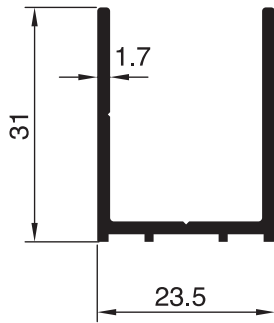
2482 - 0.384 Kg/m
