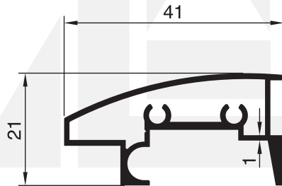
2378 - 0.448 Kg/m
