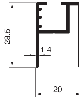
2483 - 0.365 Kg/m
