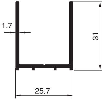
2505 - 0.393 Kg/m
