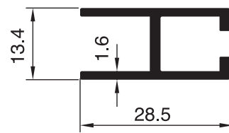
1901 - 0.330 Kg/m
