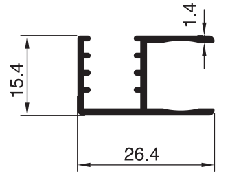
2461 - 0.263 Kg/m
