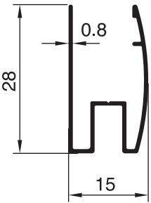
2408 - 0.192 Kg/m
