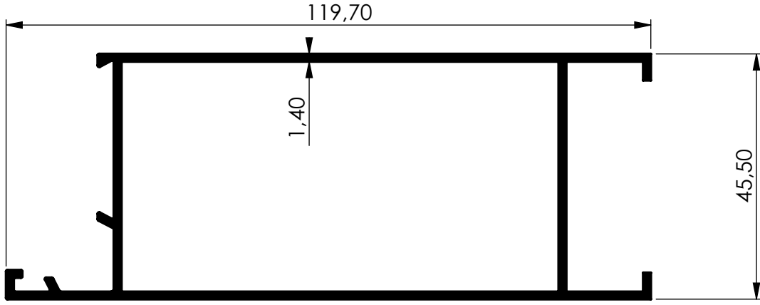
968 1.243 Kg/m 90
