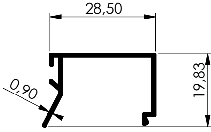
966 0.184 Kg/m
