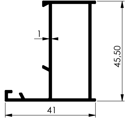
963 0.451 Kg/m
