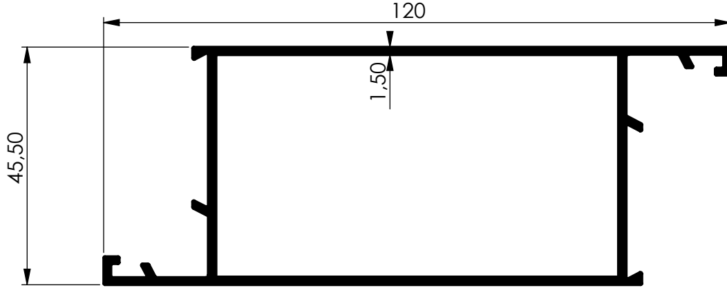
971 1.267 Kg/m
