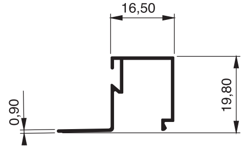
967 - 0.188 Kg/m
