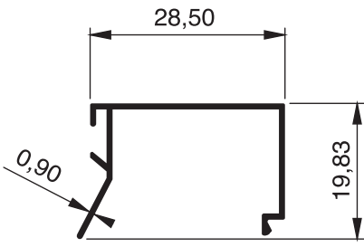
966 - 0.184 Kg/m
