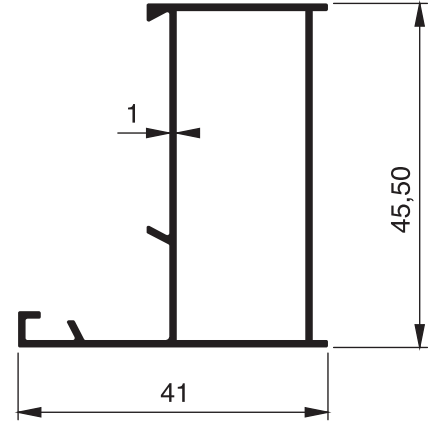
963 - 0.451 Kg/m
