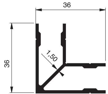
974 - 0.622 Kg/m
