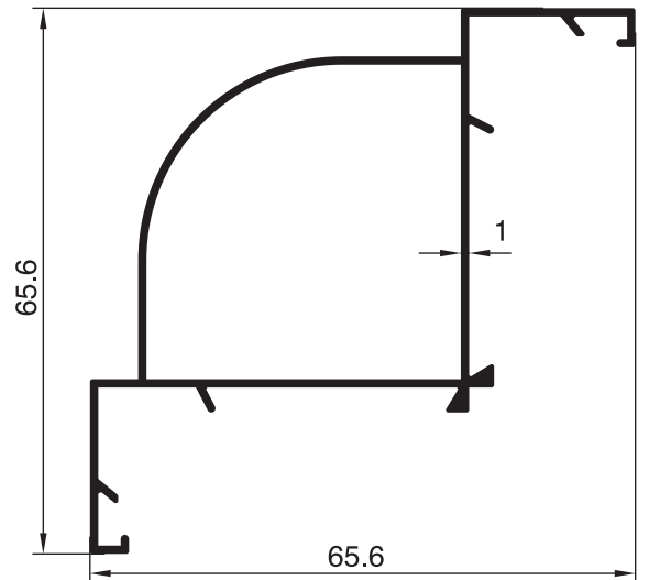
2405 - 0.628 Kg/m
