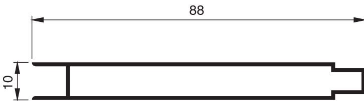
969 - 0.545 Kg/m
