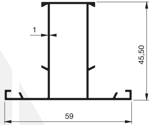
964 - 0.542 Kg/m
